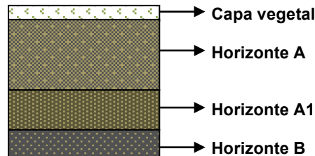
Ilustración 4. Esquema general de la estratigrafía del área sur del estudio
