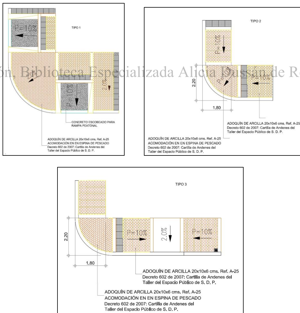
Figuras 3a, b y c. Esquema de tipos de esquinas que fueron desarrollados en las obras. Fuente: Consorcio Gama, 2015.
