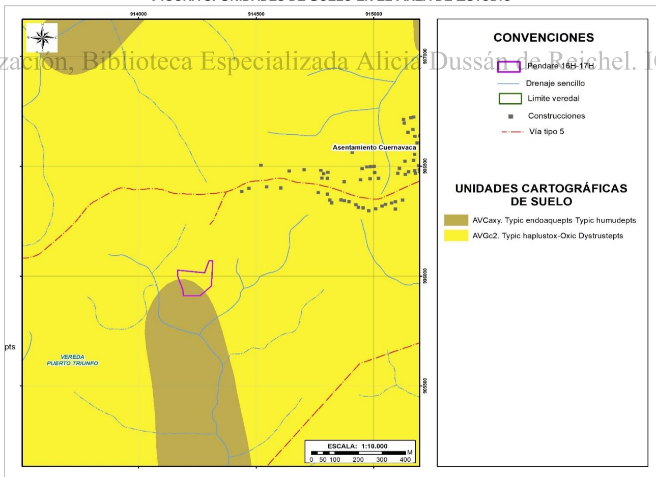
FIGURA 3. UNIDADES DE SUELO EN EL ÁREA DE ESTUDIO
